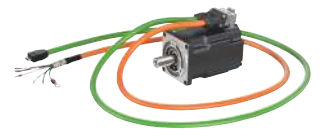
1FL2 motor MC 350 kablo DE
